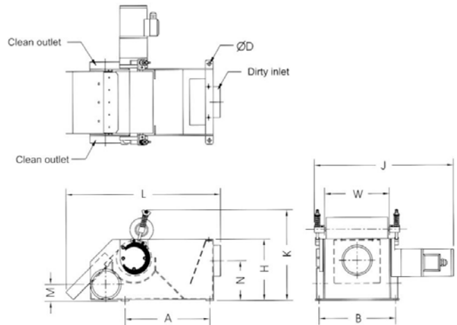
MCJ-240A Drawing
