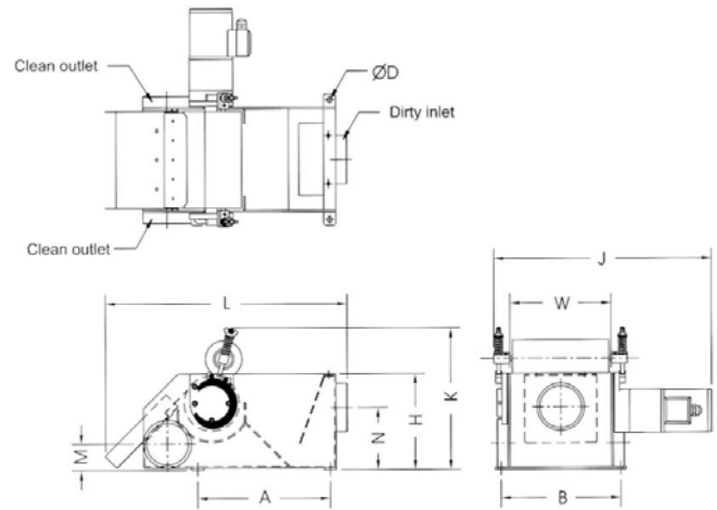
MCJ-240A Drawing
